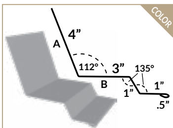
ENDWALL
