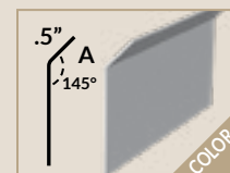
CAULK EDGE
