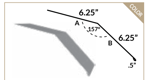
GAMBREL
